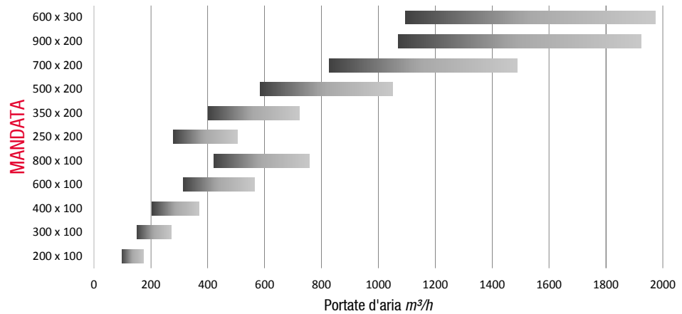
Diagramma di scelta rapida AL.VE - AL.OE
